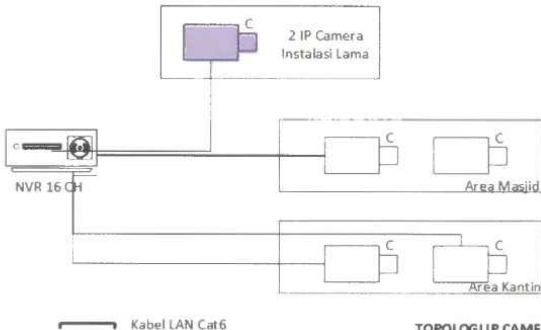
TOPOLOGI IP CAMERA Masjid dan Kantin
